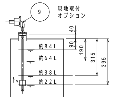
液面制御レベル図 *オプション
