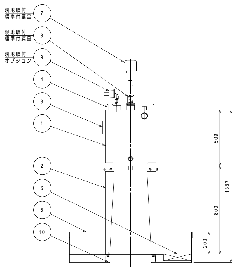
組立図
