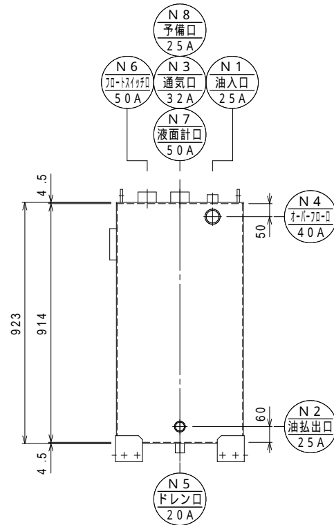
タンクノズル図
