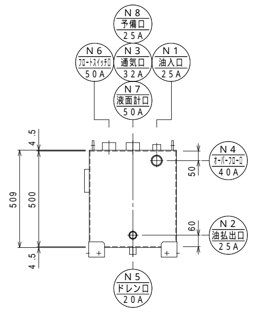
タンクノズル図
