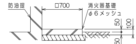
消火器基礎詳細 S: 1/40
