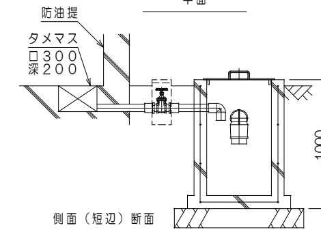
油水分離槽詳細 S: 1/40
