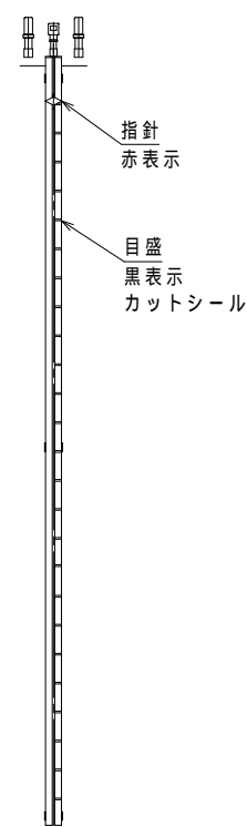
液面計正面図 S: 1/50
