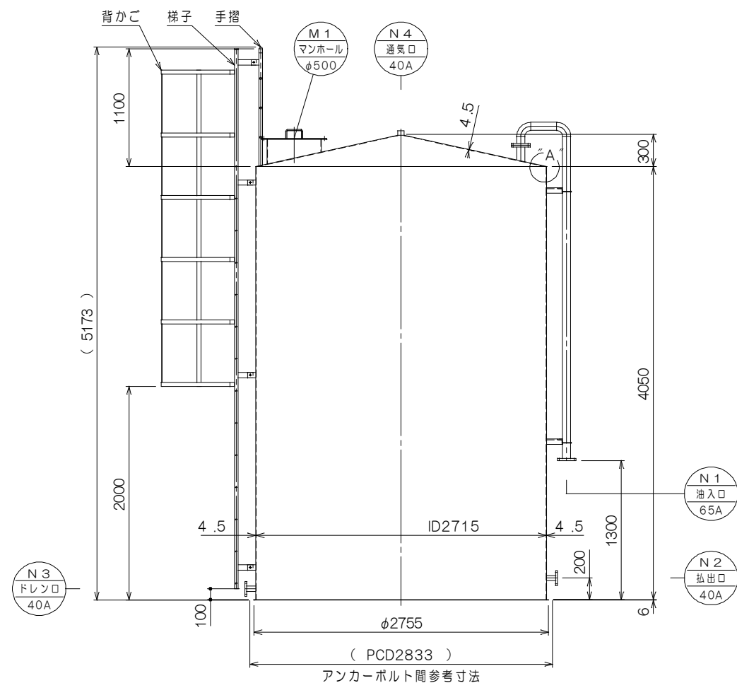
液面計正面図 S:1/50
