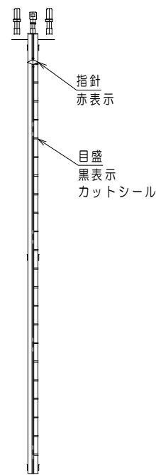
液面計正面図 S:1/50
