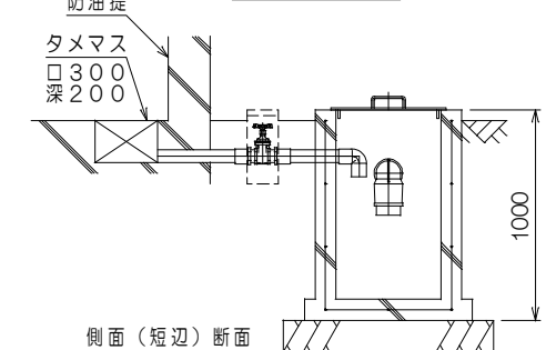
油水分離槽詳細 S: 1/40
