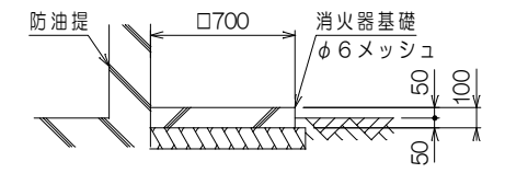
消火器基礎詳細 S: 1/40
