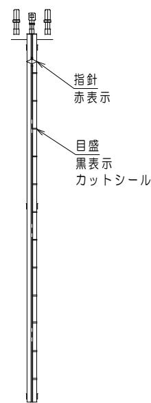
液面計正面図 S: 1/50
