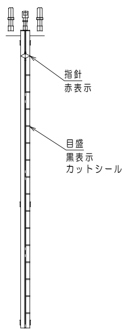
液面計正面図 S: 1/40
