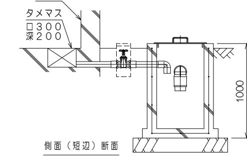
油水分離槽詳細 S: 1/40
