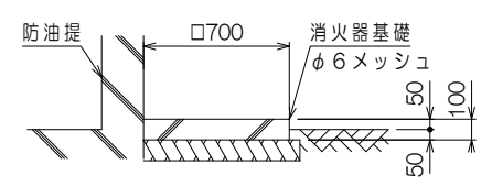
消火器基礎詳細 S: 1/40
