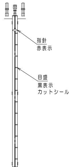
液面計正面図 S: 1/40
