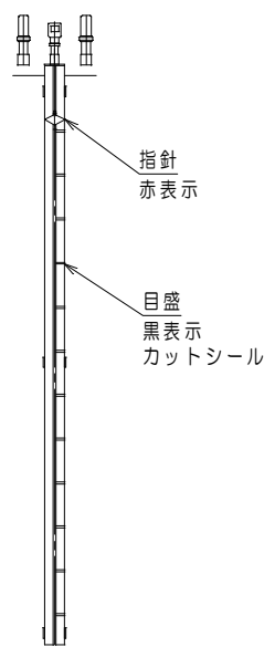
液面計正面図 S: 1/40
