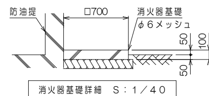
消火器基礎詳細 S: 1/40
