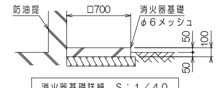
消火器基礎詳細 S: 1/40
