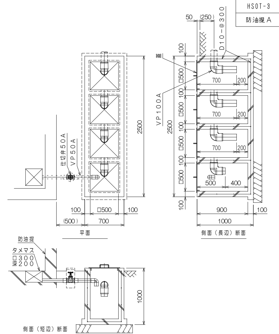
油水分離槽詳細 S: 1/40
