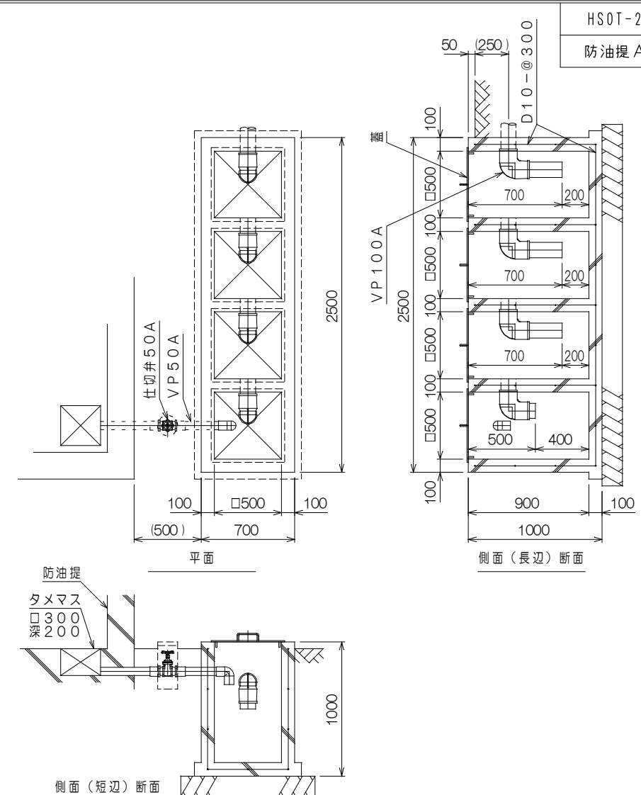
油水分離槽詳細 S: 1/40
